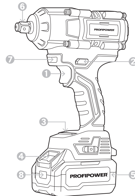
Рисунок 1.1. Устройство инструмента
